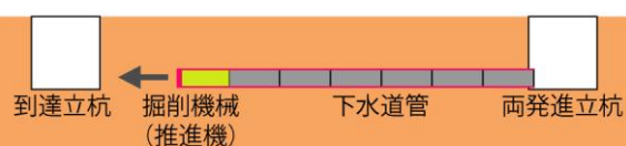
下水道工事（推進工法）のイメージ図
